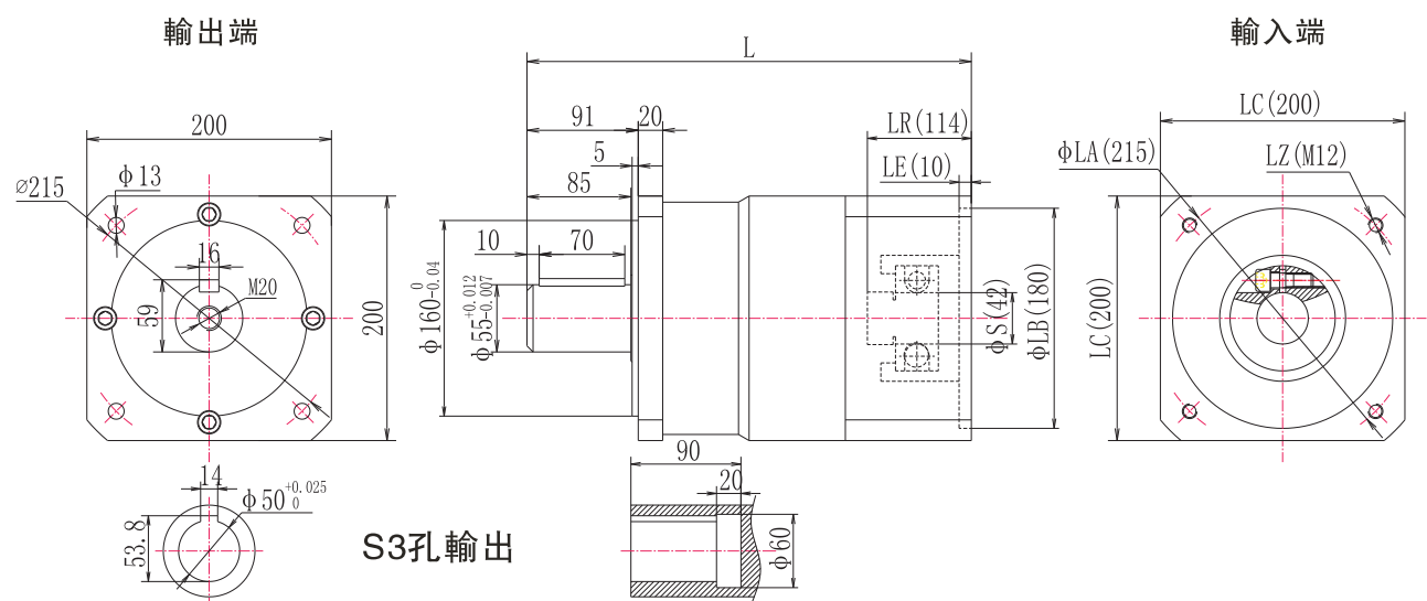
KF200外形圖
